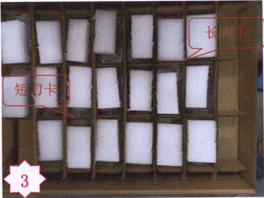
图三, 将 PA503 按照每层 120 个, 每箱三层的方式包装, 同时在底部和每层的顶部各放一块隔板, 共 4 块隔板。
